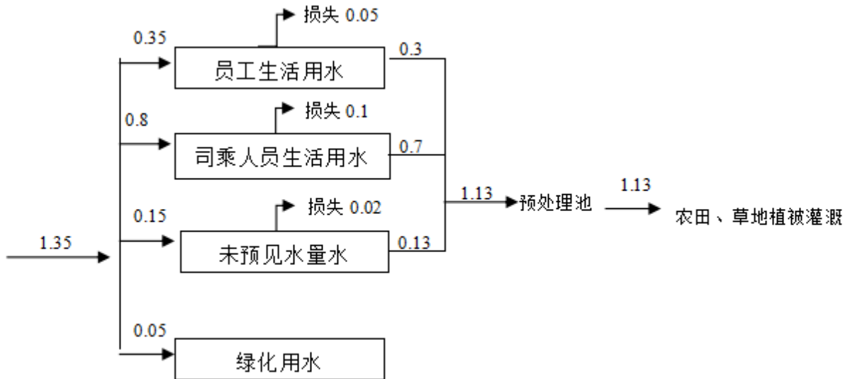
图 2-1 本项目水平衡图 单位：t/d
